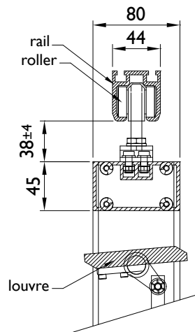
Côté haut
